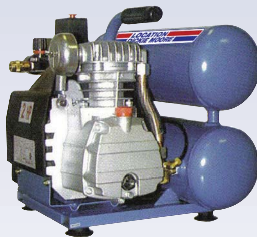
D Compresseur - Électrique - 2 CV
